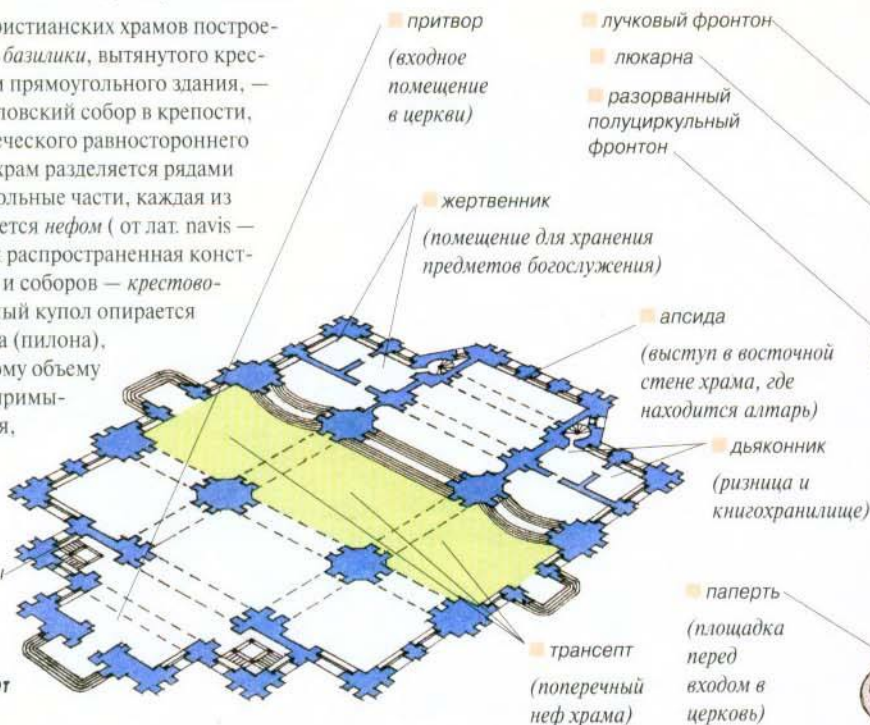
План Петропавловского собора — трехнефной базилики
